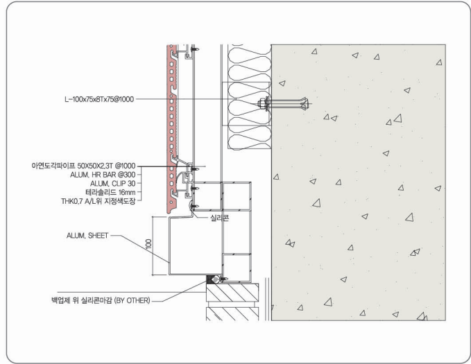
■ 외벽 하부 단면상세도
