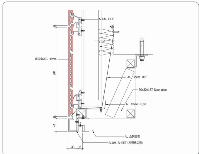
■ 정면 돌출부위 하부 단면상세도
