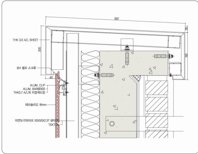
■ 파라펫 단면상세도
