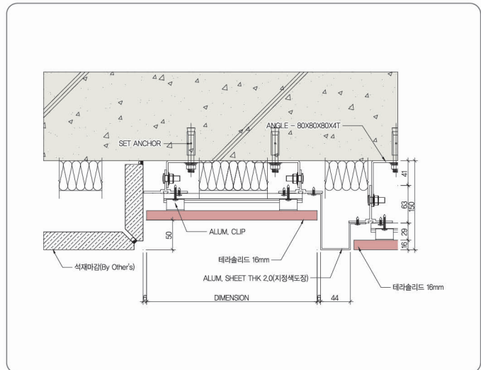
■ 이질재 접합부의 평면상세도
